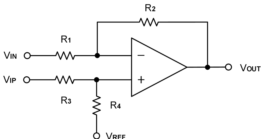
图 4. 差分放大器
